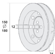
Disco Metálico con Espiga
