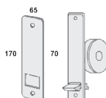
Recojedor Milán con placa de embutir
